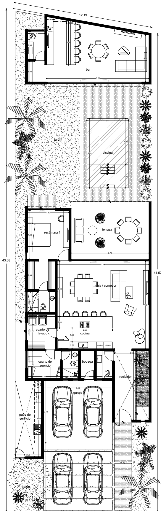
PLANTA BAJA ÁREA: 275.59m 2
